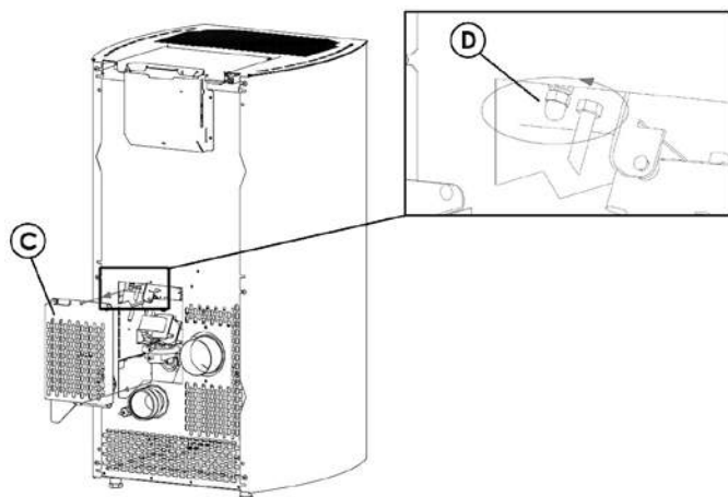
Fig. 27 - Abnehmen der Inspektionsabdeckung
