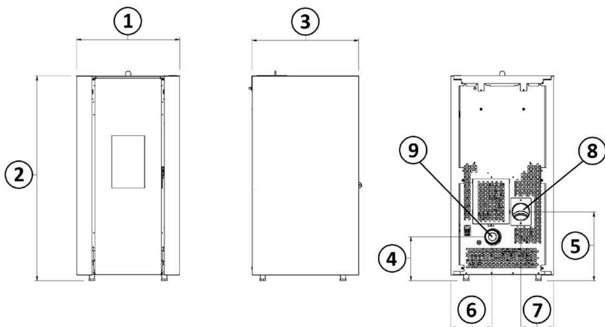
Fig. 16 - Allgemeine Abmessungen: ELANE
