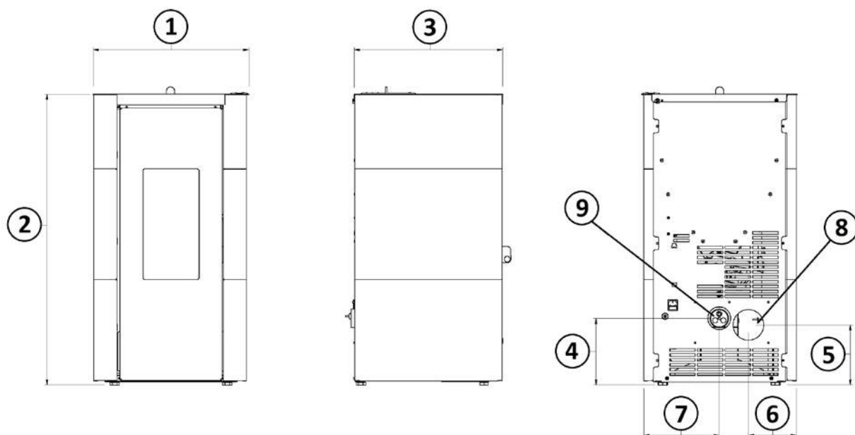
Fig. 15 - Allgemeine Abmessungen: TALAS³
