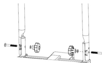
Figura 2: Montaggio staffa a U
