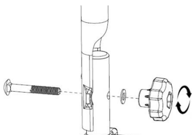
Figure 3 : Fixation de l'étrier en U
