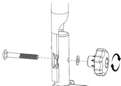
Bild 3: Festschrauben U-Bügel
