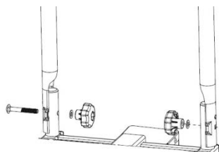
Obrázek 2: Montážní U-konzola
