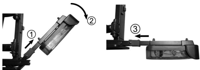
Figure 12 : Verrouillage du support d'éclairage
