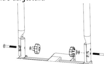
Bild 2: Montage U-Bügel
