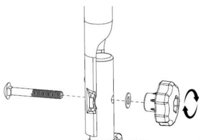
Obrázek 3: Utahování U-konzoly
